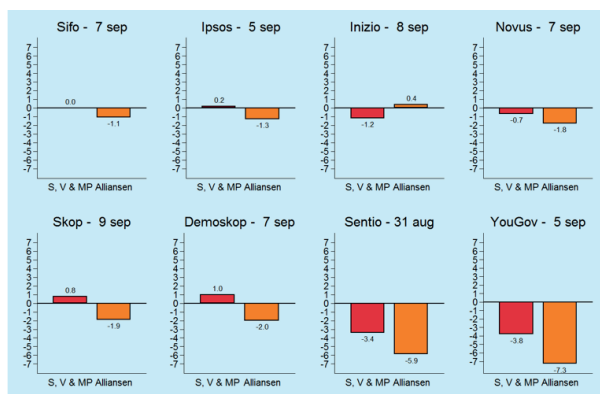
Figur 3. Över och underskattningar på blocknivå inför 2018 års riksdagsval (procentenheter)
