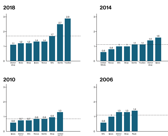
Figur 1. Genomsnittlig avvikelse för respektive opinionsinstitut och år (procentenheter)
